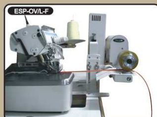
스파게티용 감속기 (롤러 폭 : 上 50mm, 下 60mm) 디지털 감속기이며, 회전 8,500RPM까지 사용가능합니다. 오바, 인터, 본봉에 사용가능하며, 타 기종에도 적용가능합니다. FOR SPAGHETTI
